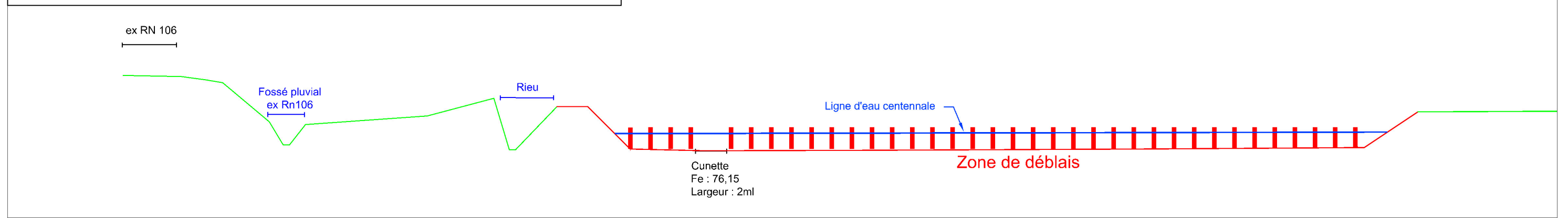
Profil en travers au droit de la zone d'implantation du peigne à embâcles
